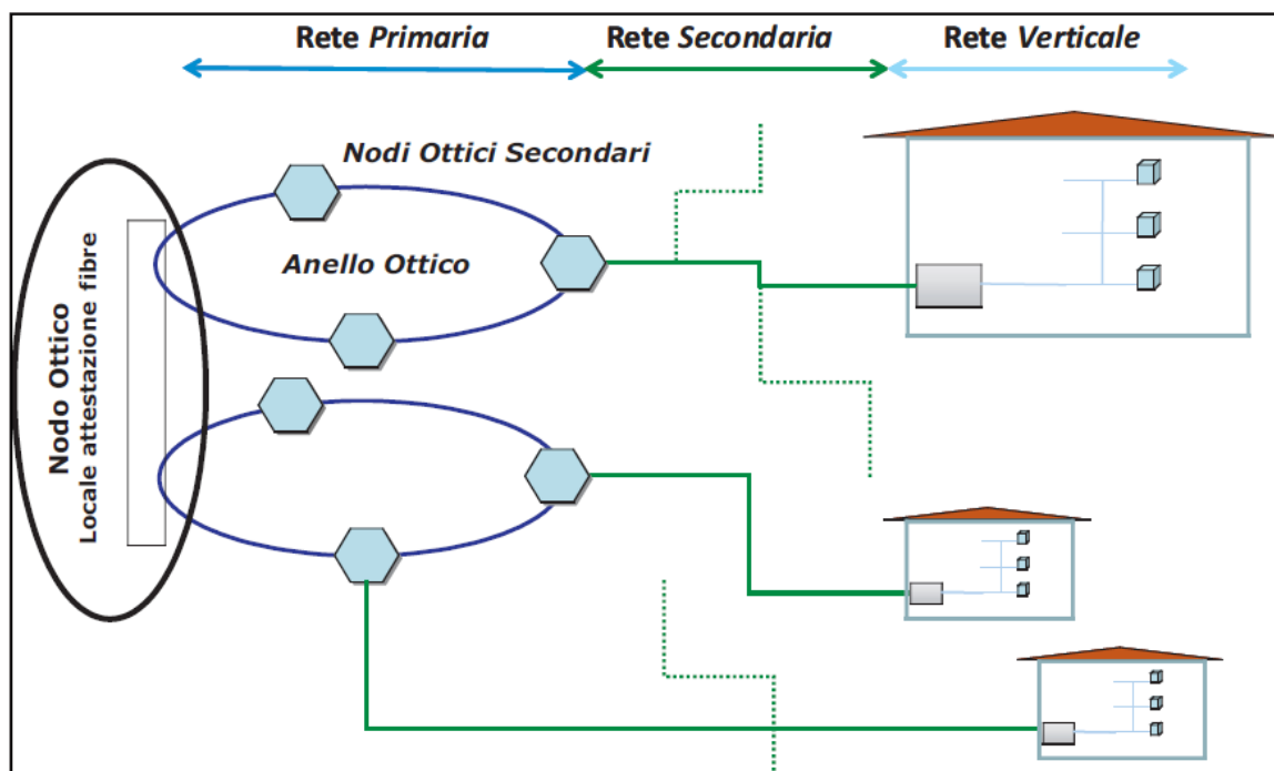
Figura 11 – Architettura tecnica di riferimento
